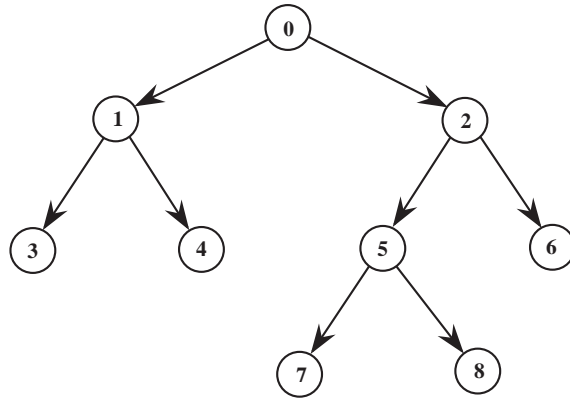
Fig. 9.1.1 Albero di enumerazione.
