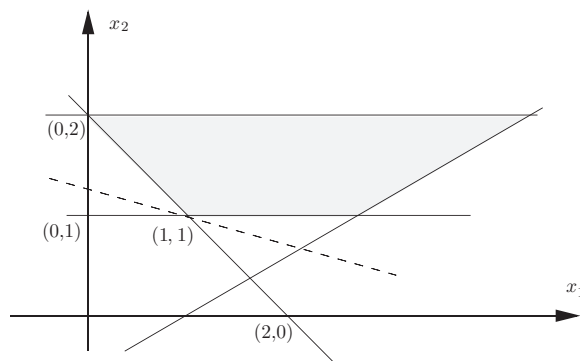
Fig. 9.1.4 Soluzione grafica del Problema Prob^{(4)} dell'Esercizio 9.1.3.
