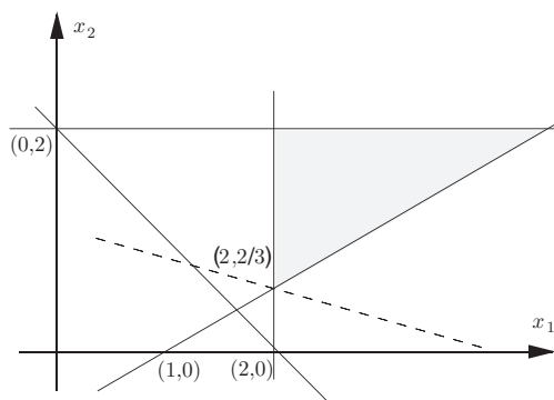
Fig. 9.1.3 Soluzione grafica del Problema Prob^{(2)} dell'Esercizio 9.1.3.
