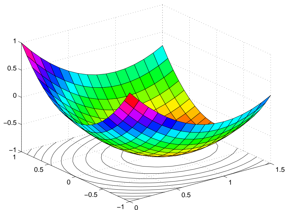
Figure 3.6: Grafico di q(x_1, x_2) per \alpha = \beta = 1 .
